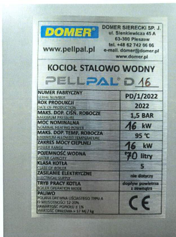
Rysunek 12 Tabliczka znamionowa
