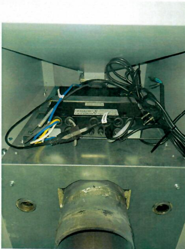
Rysunek 10 Moduł Sterownika PELLPAL PLUS firmy ProND
