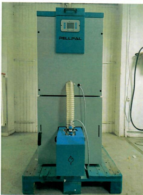
Rysunek 2 Badany kotł
