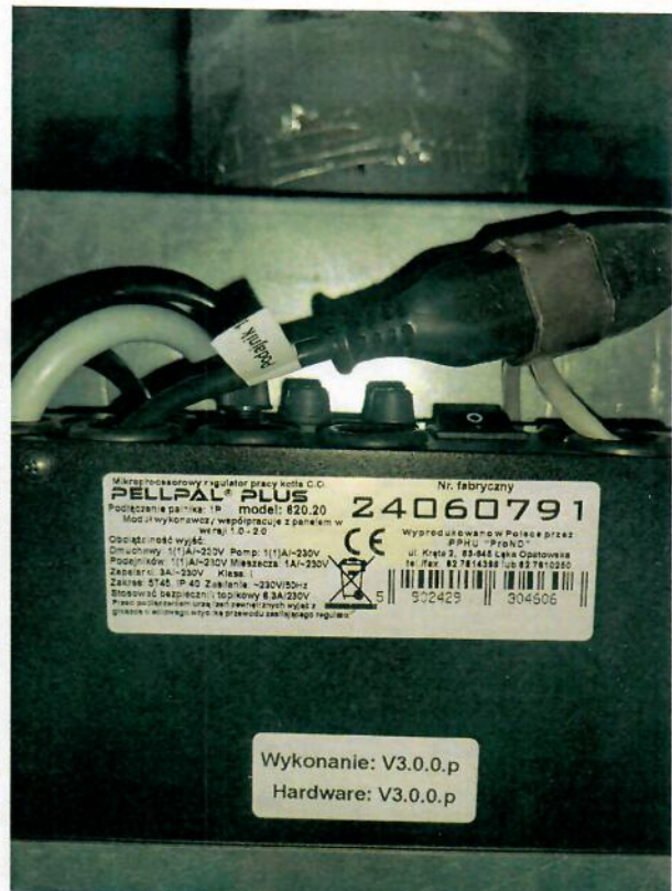
Rysunek 11 Moduł Sterownika PELLPAL PLUS firmy ProND
