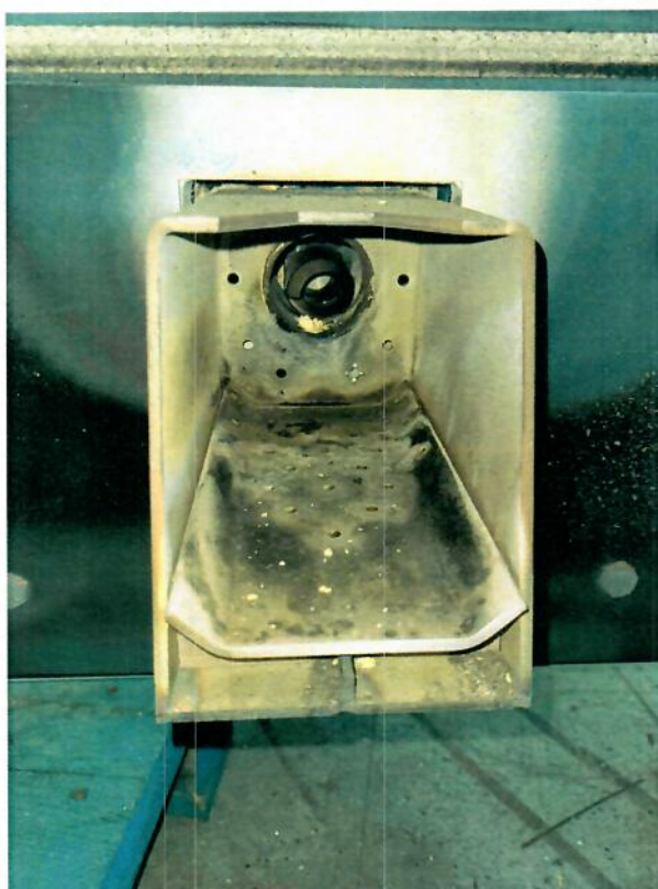
Rysunek 6 Palnik
